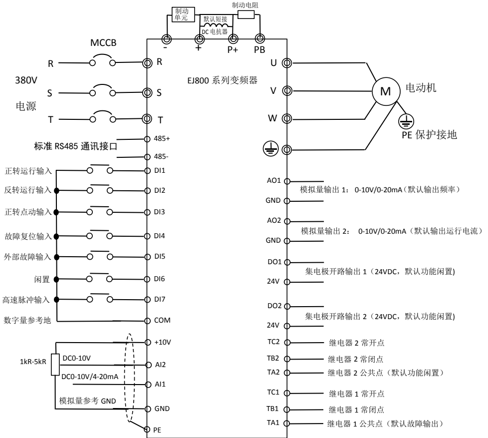
图 3.2 基本运行配线图
